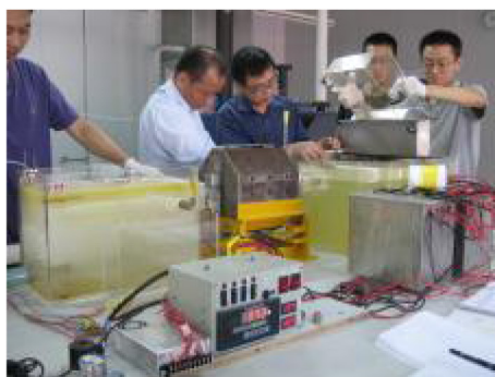
循环回路油水分离装置
