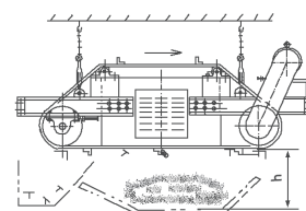
安装示意图（水平式）
