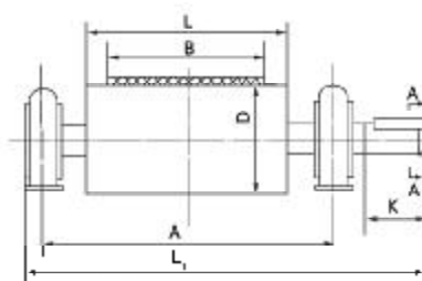
外形尺寸图
