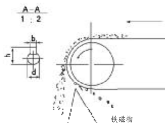
安装示意图
