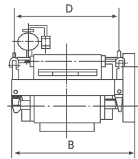
外形尺寸图
