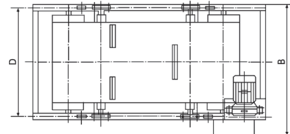
外形尺寸图
