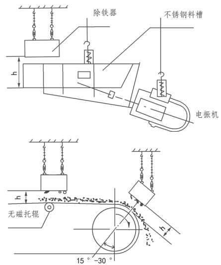
安装示意图
