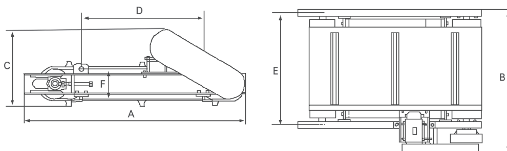
外形尺寸图
